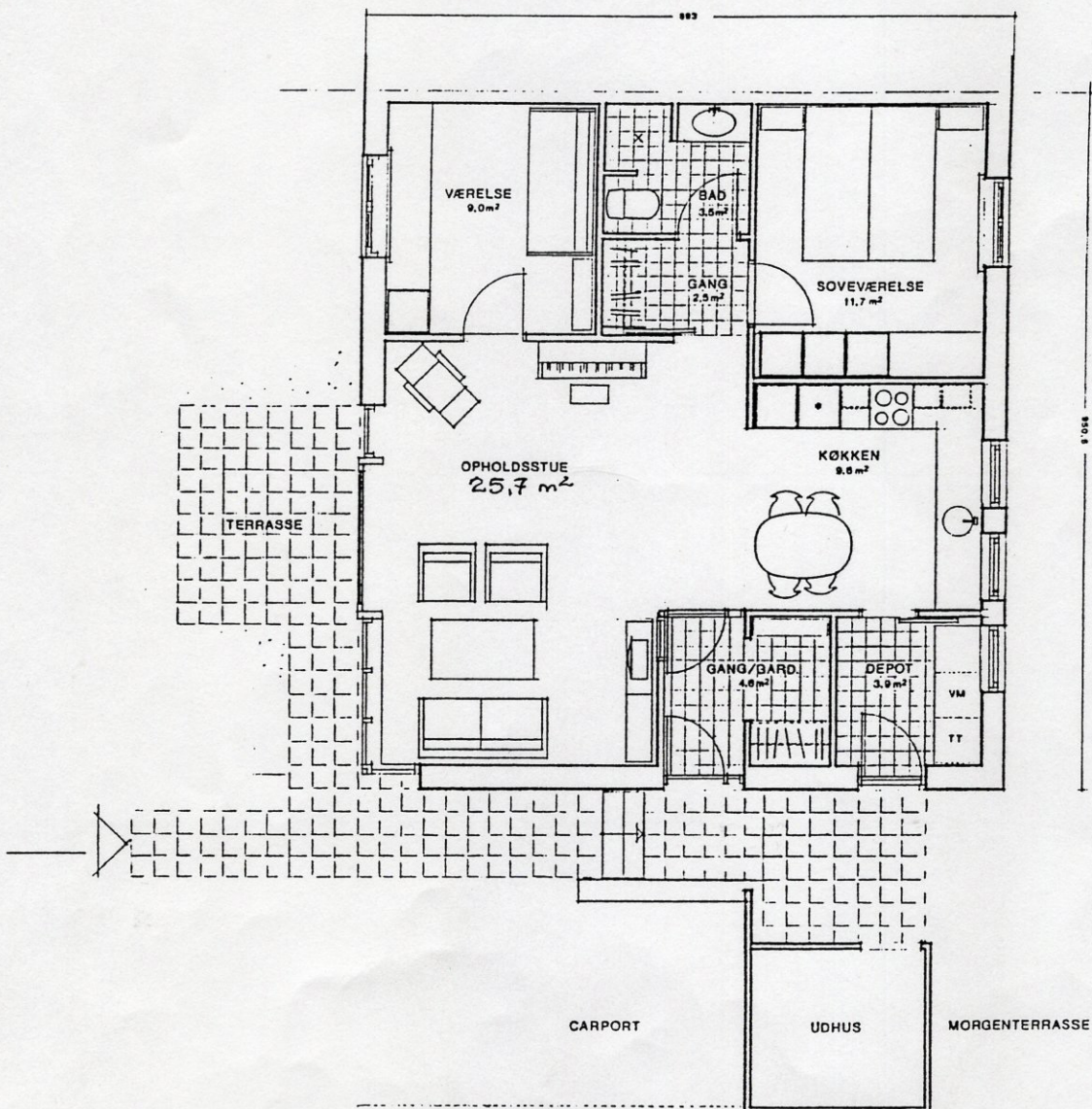
TYPE 85 · ALT I ÉT PLAN
