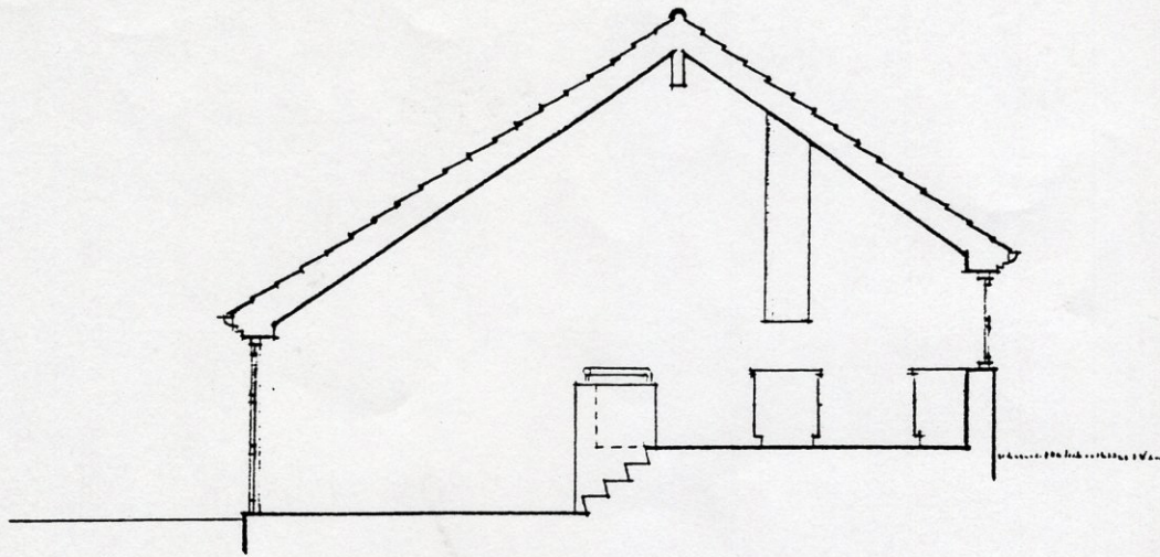
SNIT I TYPE 85 · FORSKUDT
